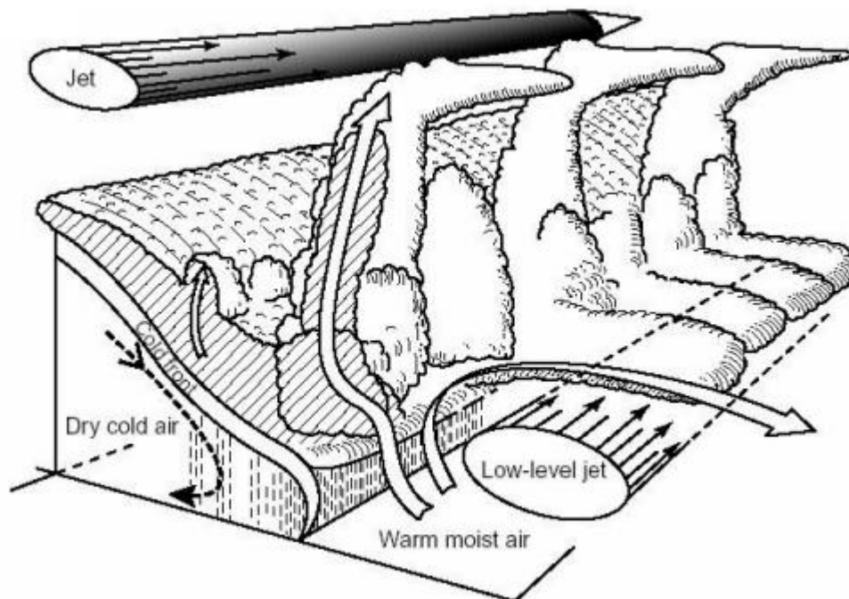
Зураг 3. Хүйтэн фронтын схем, нам өндрийн болон өндрийн олгойдох урсгал байрлал
