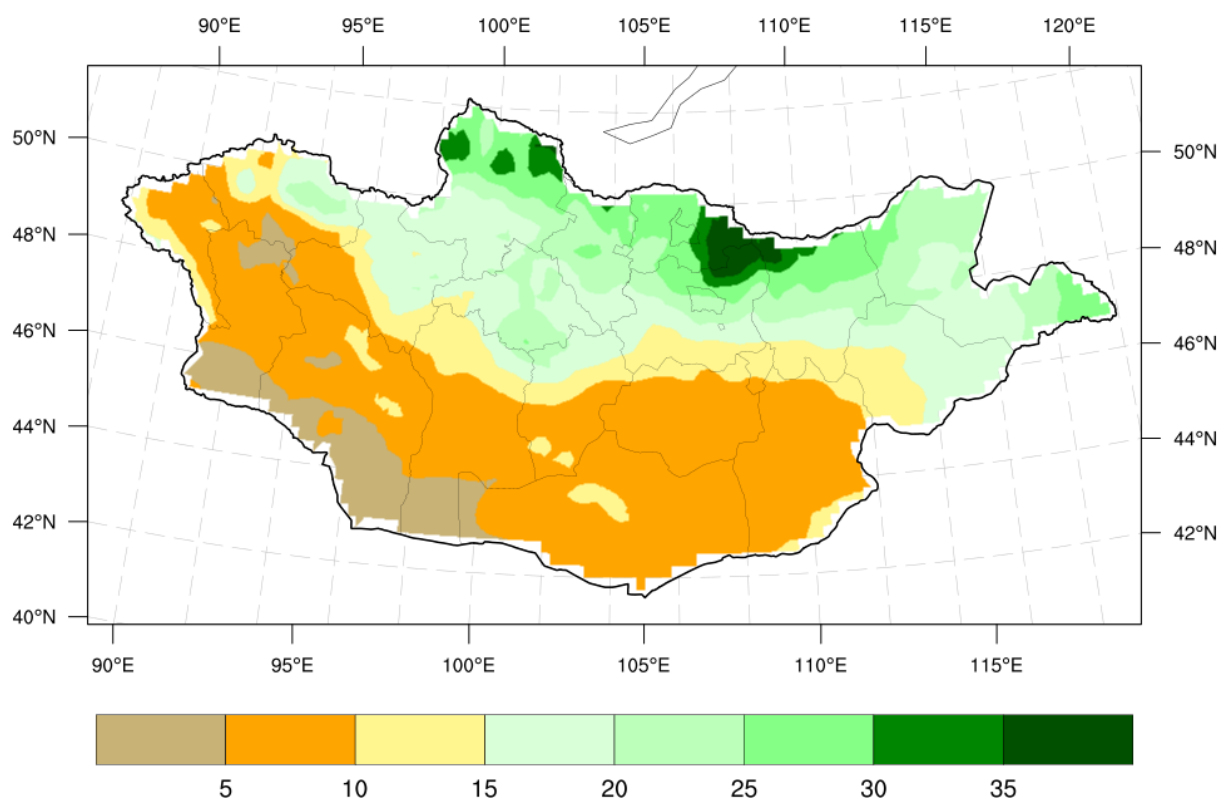
Зураг 4а. 9 дүгээр сарын хур тунадасны ОЖД (1991-2020)
