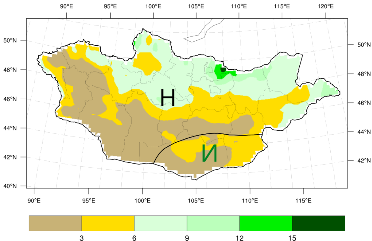
Зураг 6б. 2025 оны 10 дугаар сарын хур тунадасны урьдчилсан төлөв (мм)
