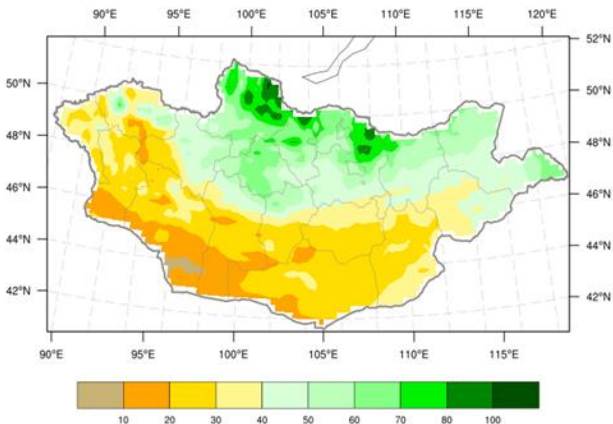
Зураг 2а. 8 дугаар сарын хур тунадасны ОЖД (1991-2020)
