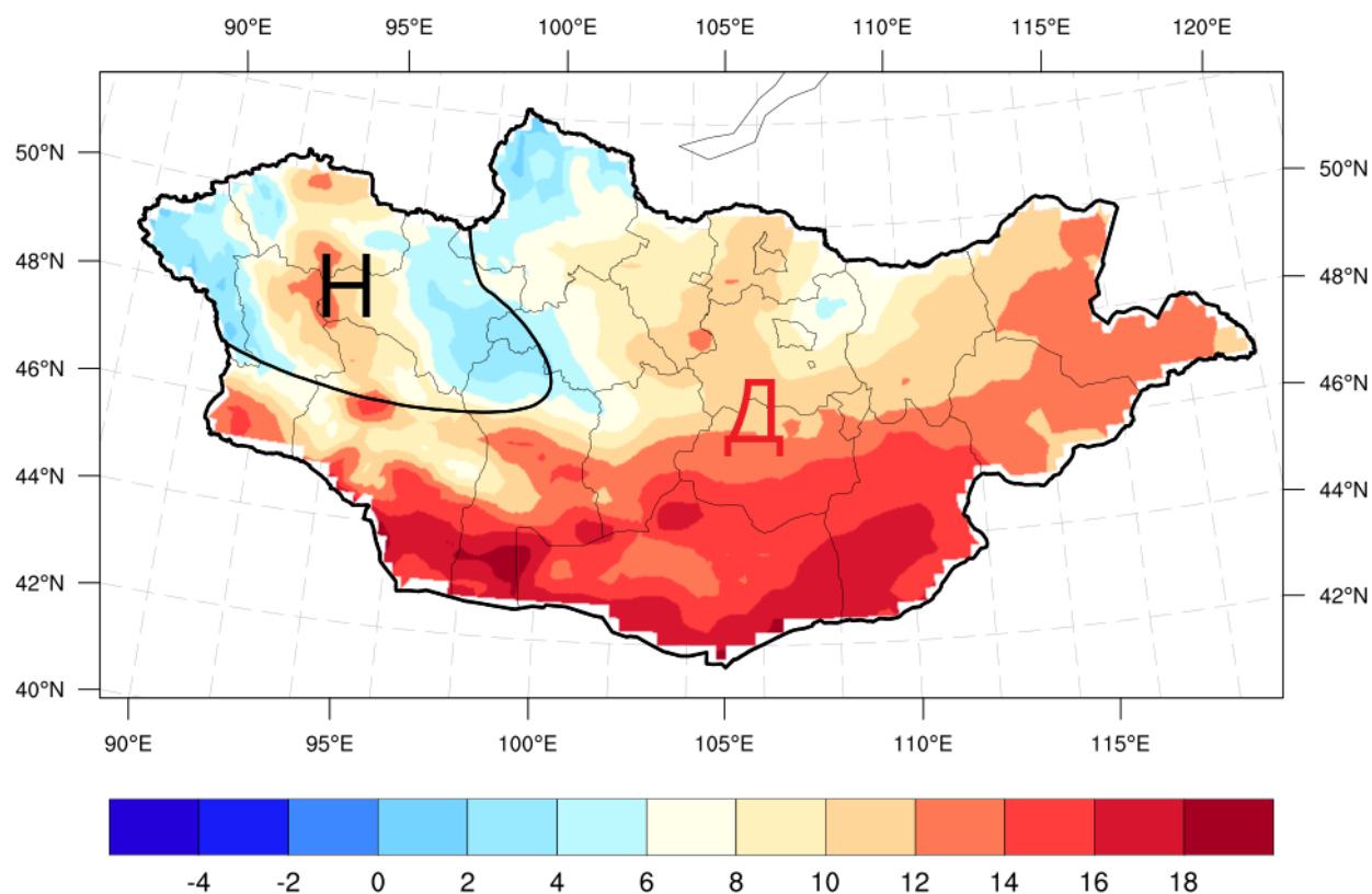
Зураг 3б. 2025 оны 9 дүгээр сарын агаарын дундаж температурын урьдчилсан төлөв (°C)
