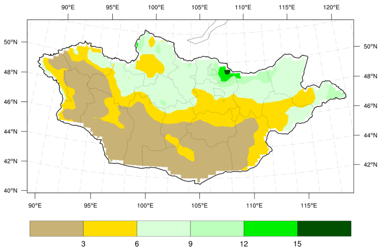
Зураг ба. 10 дугаар сарын хур тунадасны ОЖД (1991-2020)
