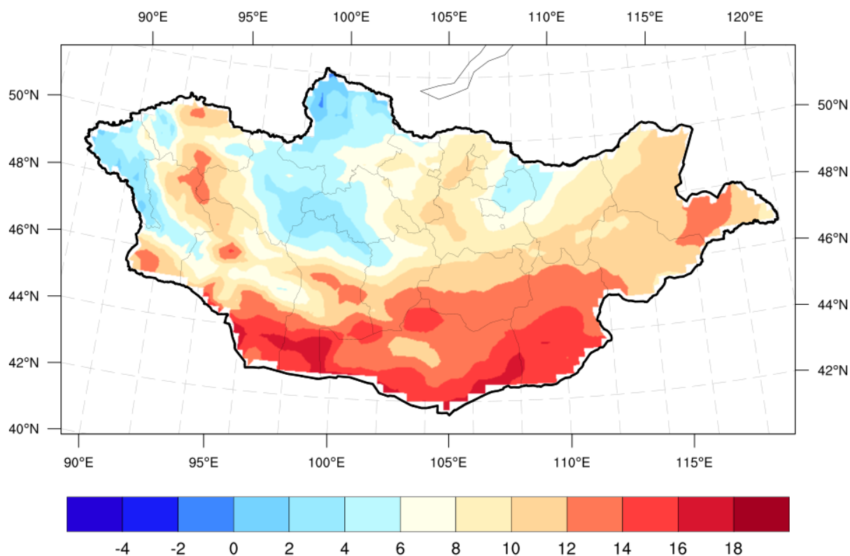
Зураг 3а. 9 дүгээр сарын агаарын дундаж температурын ОЖД (1991-2020)
