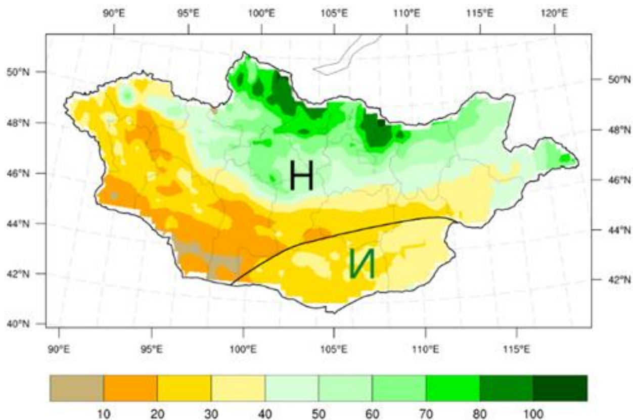
Зураг 26. 2025 оны 8 дугаар сарын хур тунадасны урьдчилсан төлөв (мм)
