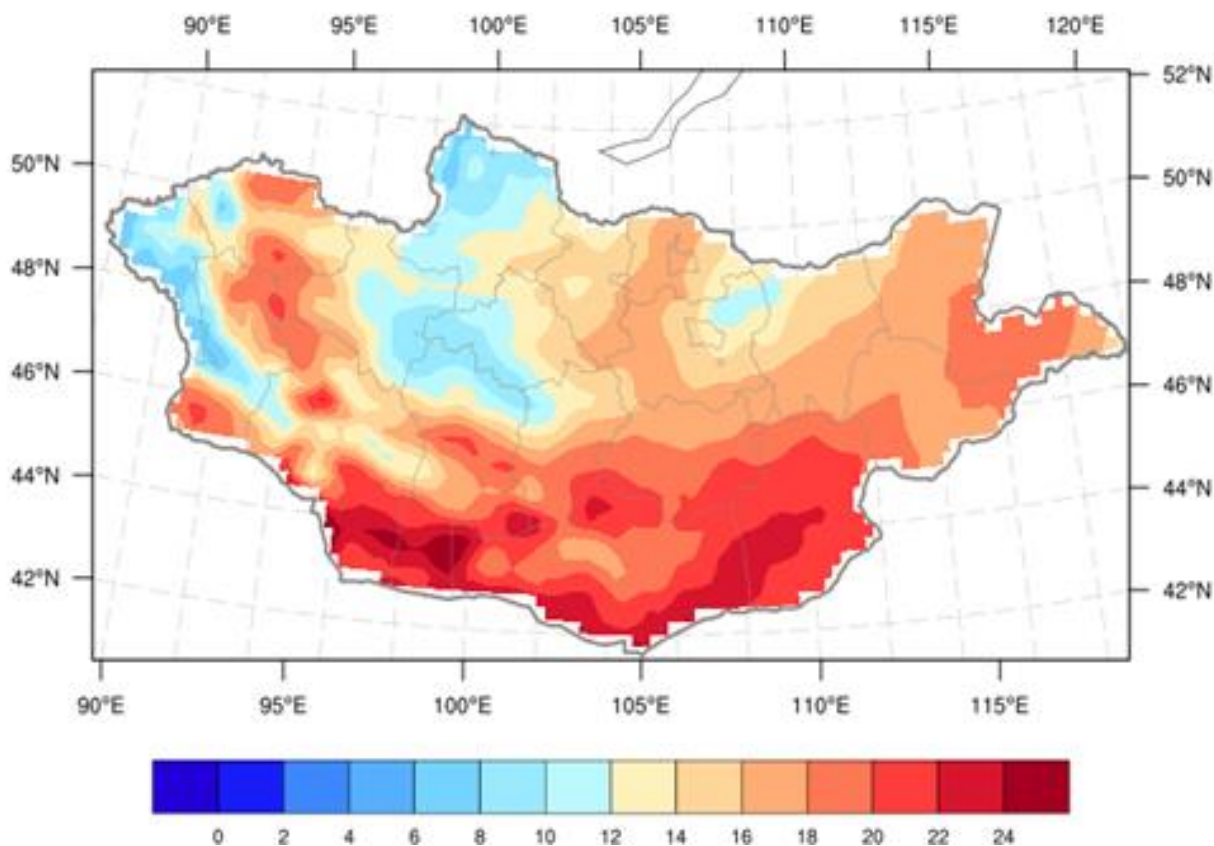
Зураг 1а. 8 дугаар сарын агаарын дундаж температурын ОЖД (1991-2020)
