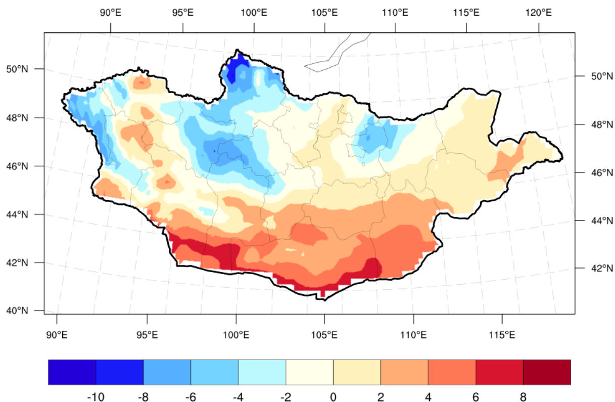
Зураг 5а. 10 дугаар сарын агаарын дундаж температурын ОЖД (1991-2020)
