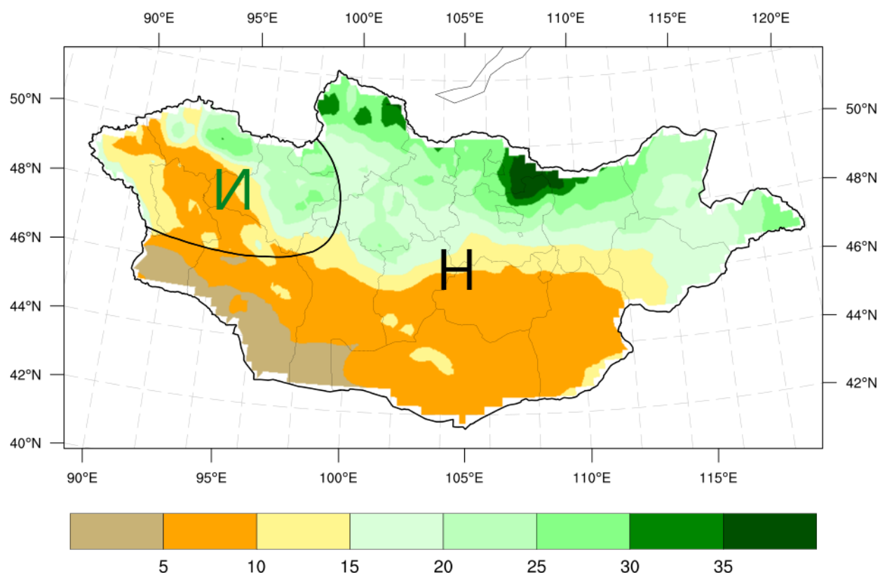
Зураг 46. 2025 оны 9 дүгээр сарын хур тунадасны урьдчилсан төлөв (мм)
