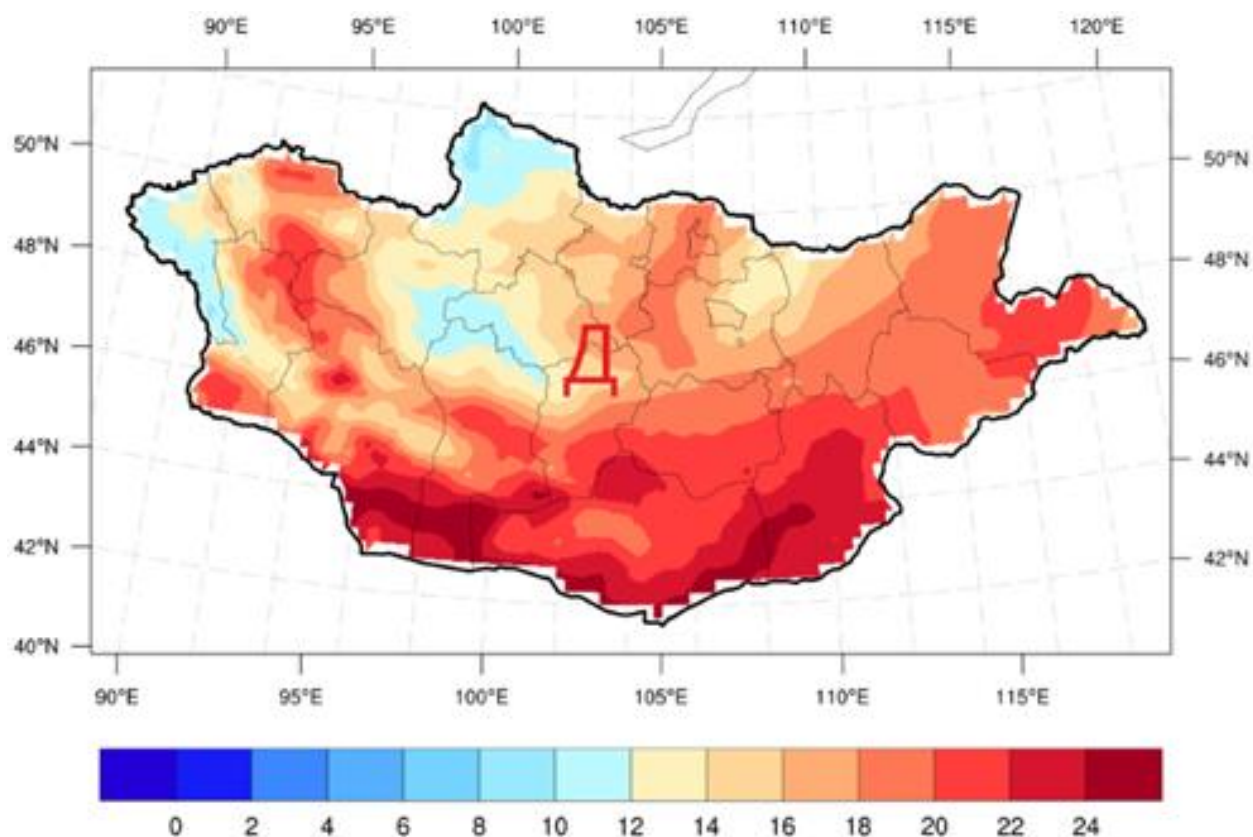
Зураг 16. 2025 оны 8 дугаар сарын агаарын дундаж температурын урьдчилсан төлөв (°C)
