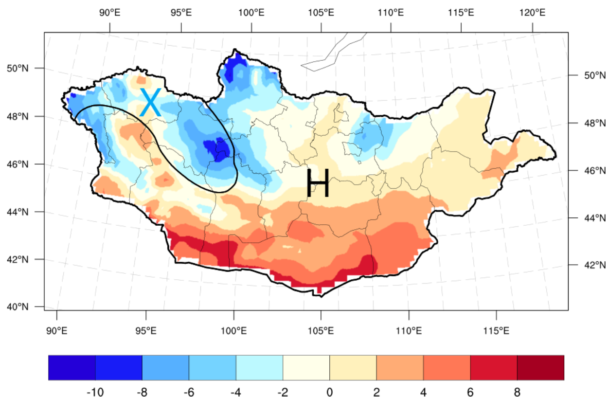
Зураг 56. 2025 оны 10 дугаар сарын агаарын дундаж температурын урьдчилсан төлөв (°C)
