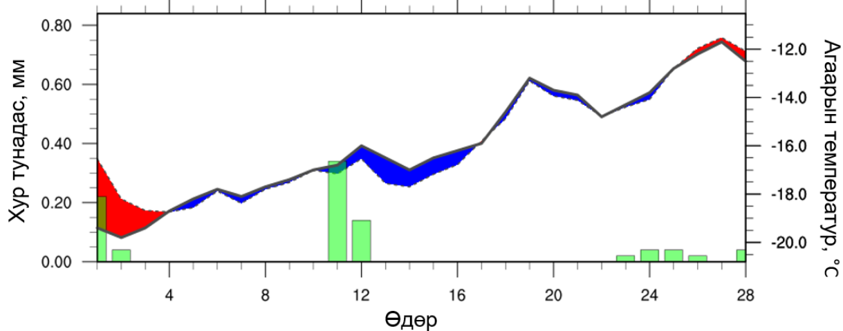
Зураг 9. Зүүн аймгуудын нутгийн 2025 оны 2-р сарын температур, хур тунадасны явц
