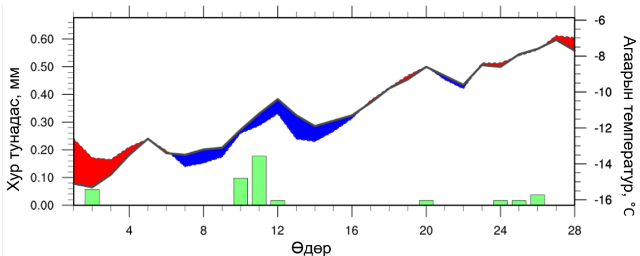
Зураг 10. Говийн аймгуудын нутгийн 2025 оны 2-р сарын температур, хур тунадасны явц [Хөх – агаарын дундаж температур ОЖД-аас хүйтэн, улаан – агаарын дундаж температур ОЖД-аас дулаан, үргэлжилсэн хар зураас – агаарын дундаж температур, тасархай хар зураас – агаарын дундаж температурын ОЖД-аас хазайх хазайц, ногоон – хур тунадасны хэмжээ]
