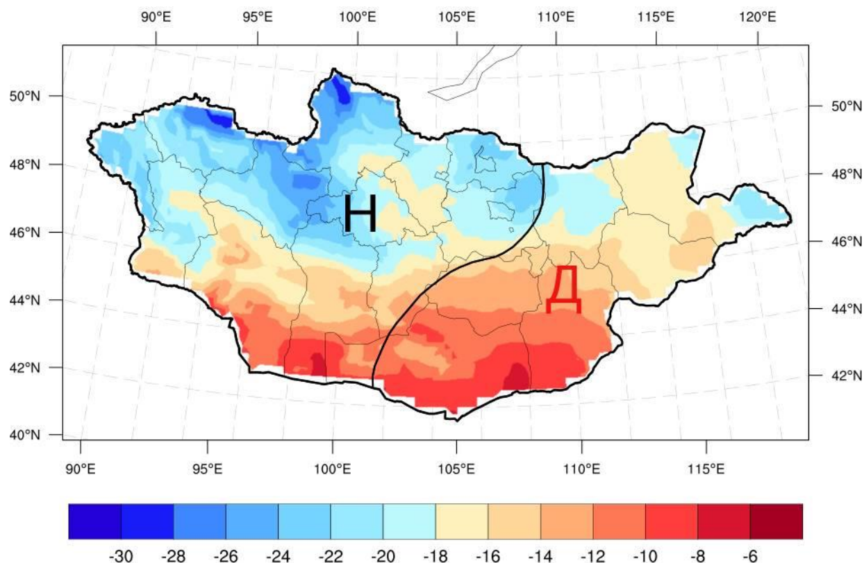
Зураг 5. 2025 оны 2-р сарын агаарын дундаж температурын урьдчилсан төлөв, С° [Д-агаарын температур ОЖД–аас дулаан, Н-агаарын температур ОЖД–ийн орчим]
