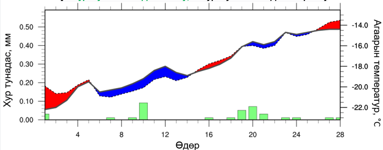
Зураг 7. Баруун аймгуудын нутгийн 2025 оны 2-р сарын температур, хур тунадасны явц [Хөх – агаарын дундаж температур ОЖД-аас хүйтэн, улаан – агаарын дундаж температур ОЖД-аас дулаан, үргэлжилсэн хар зураас – агаарын дундаж температур, тасархай хар зураас – агаарын дундаж температурын ОЖД-аас хазайх хазайц, ногоон – хур тунадасны хэмжээ]
