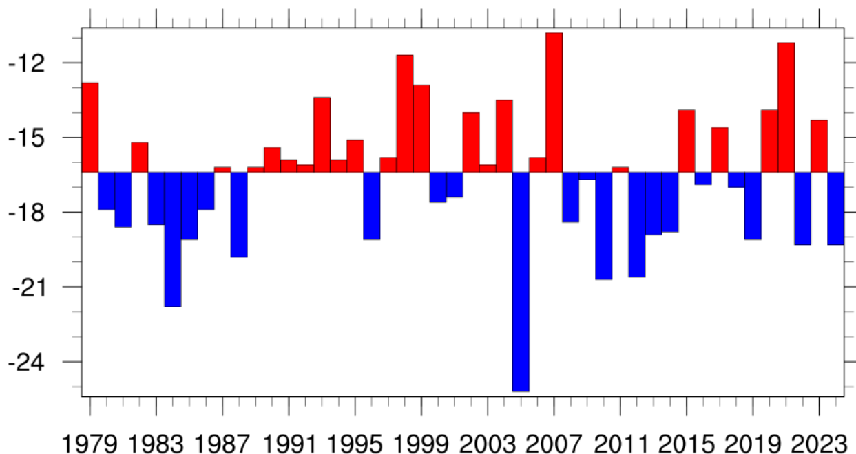
Зураг 2. 2-р сарын агаарын температурын олон жилийн явц [Улаан – ОЖД-аас дулаан, хөх – ОЖД-аас хүйтэн]
