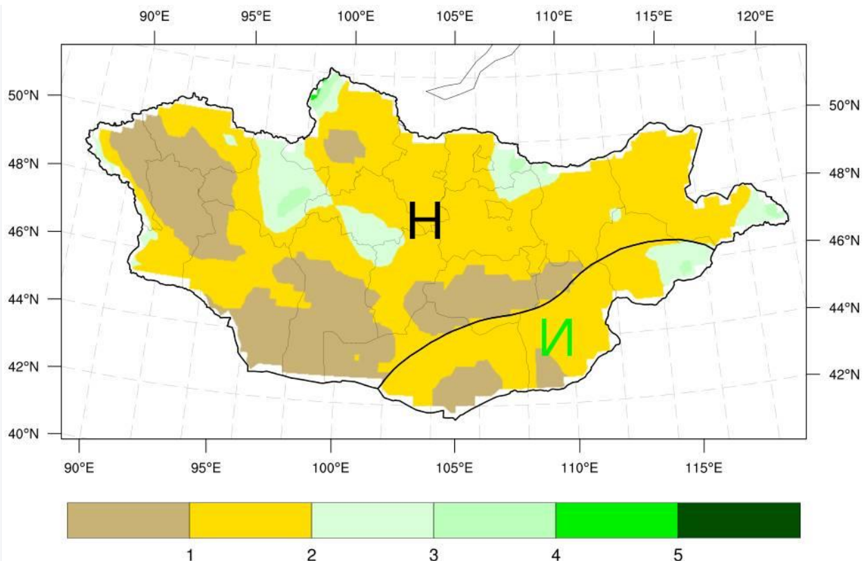
Зураг 6. 2025 оны 2-р сарын нийлбэр хур тунадасны урьдчилсан төлөв, мм [И-хур тунадас ОЖД-аас ахиу, Н-хур тунадас ОЖД-ийн орчим]
