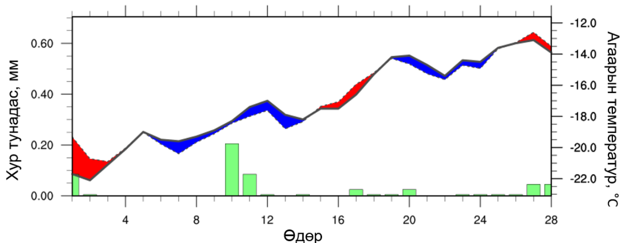
Зураг 8. Төвийн аймгуудын нутгийн 2025 оны 2-р сарын температур, хур тунадасны явц
