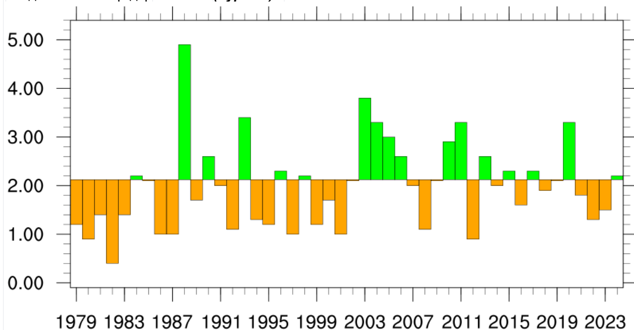
Зураг 4. 2-р сарын нийлбэр хур тунадасны олон жилийн явц [Ногоон – ОЖД-аас ахиу, шар – ОЖД-аас бага]
