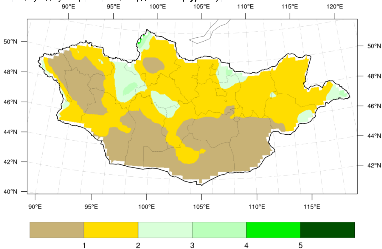
Зураг 3. 2-р сарын нийлбэр хур тунадасны ОЖД, [мм]
