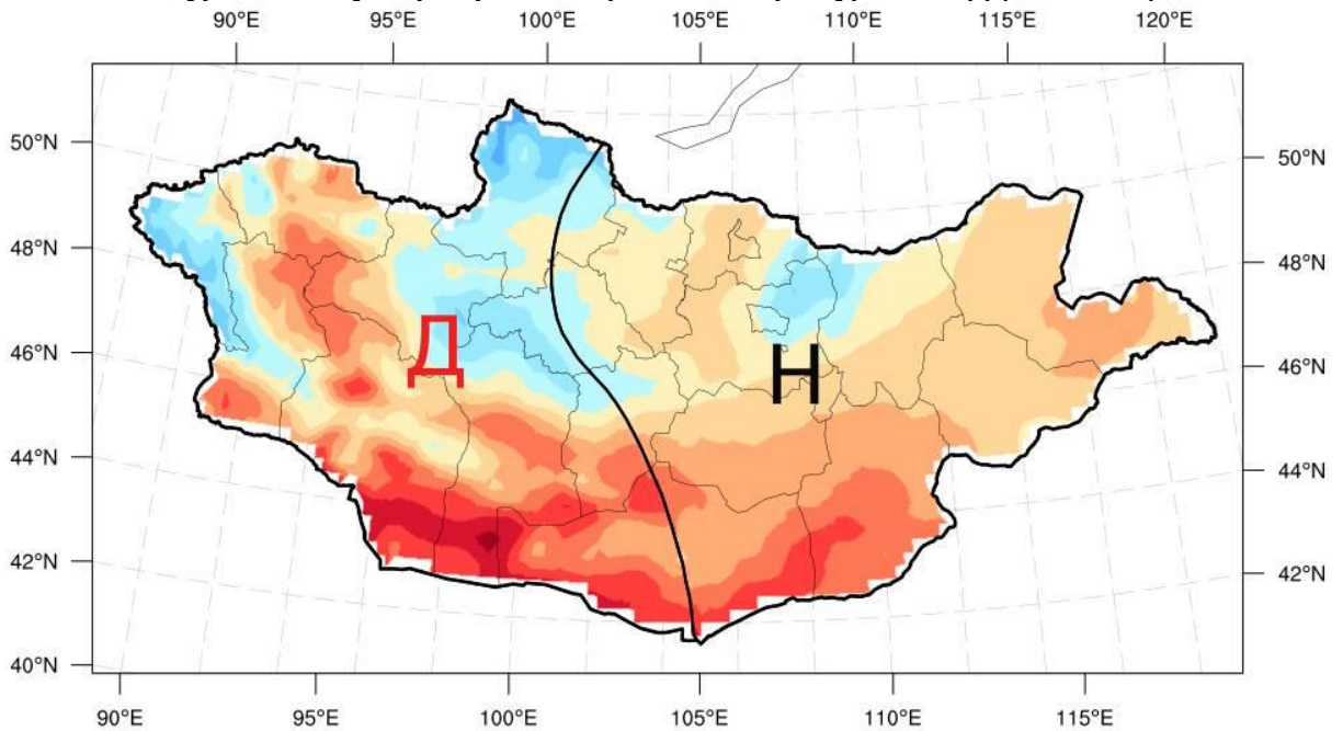
Зураг 1а. 5 дугаар сарын агаарын температурын ОЖД (1991-2020)
