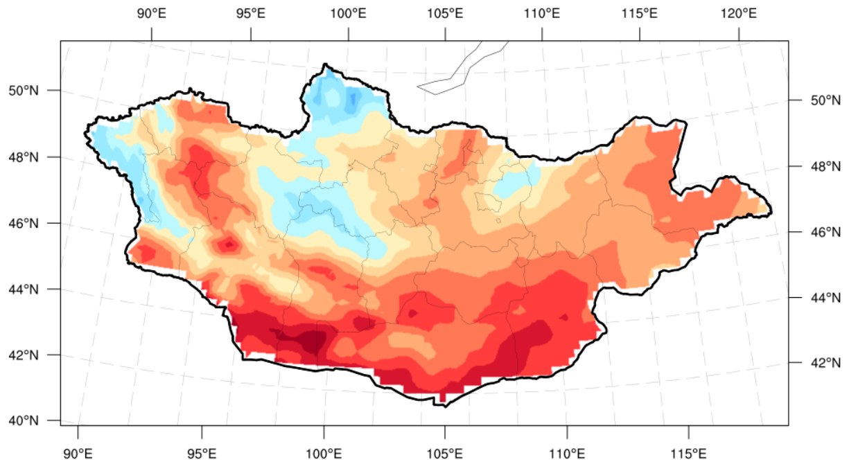
Зураг 3а. 6 дугаар сарын агаарын температурын ОЖД (1991-2020)
