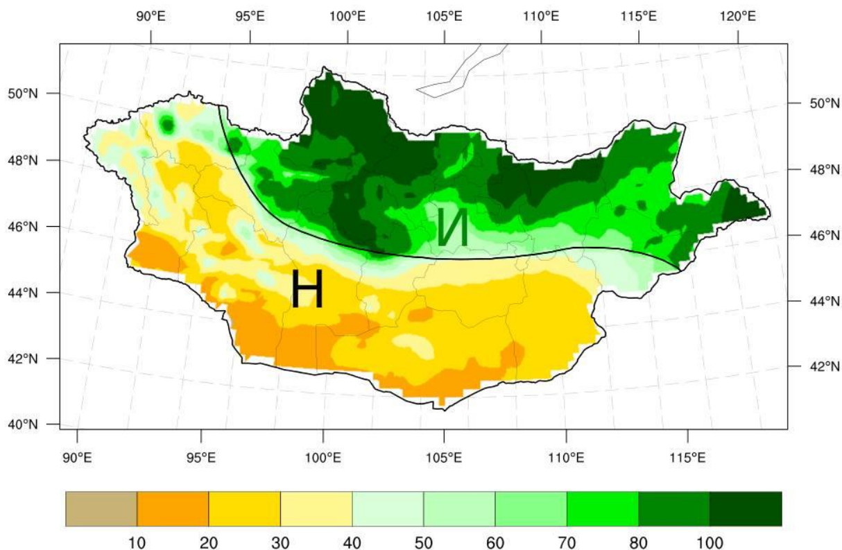
Зураг 6б. 2024 оны 7 дугаар сарын хур тунадасны урьдчилсан төлөв (мм) [Н-хур тунадас ОЖД-ийн орчим, И-хур тунадас ОЖД-аас ахиу]
