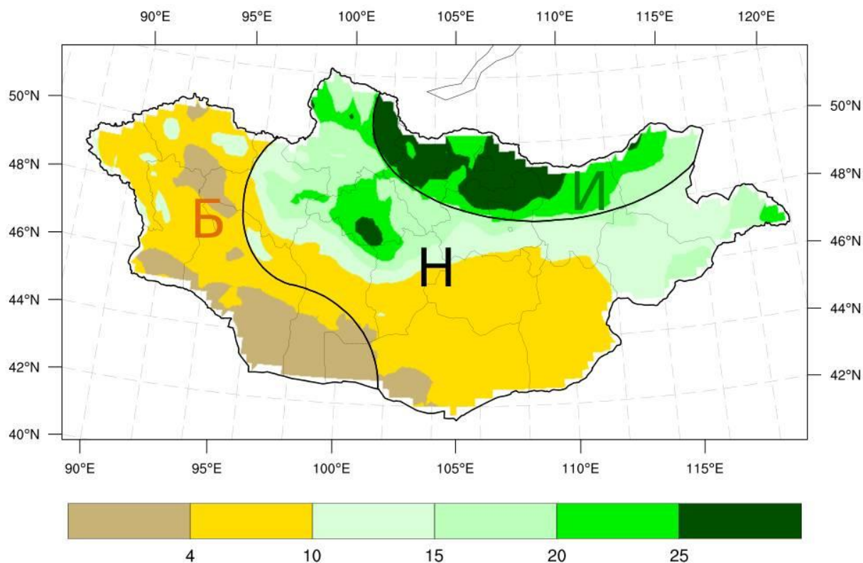
Зураг 26. 2024 оны 5 дугаар сарын хур тунадасны урьдчилсан төлөв (мм)
