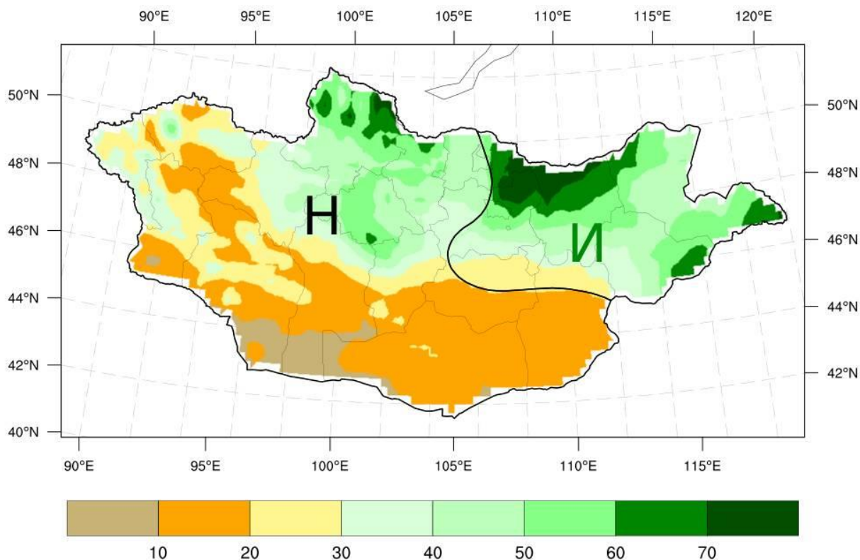
Зураг 46. 2024 оны 6 дугаар сарын хур тунадасны урьдчилсан төлөв (мм)
