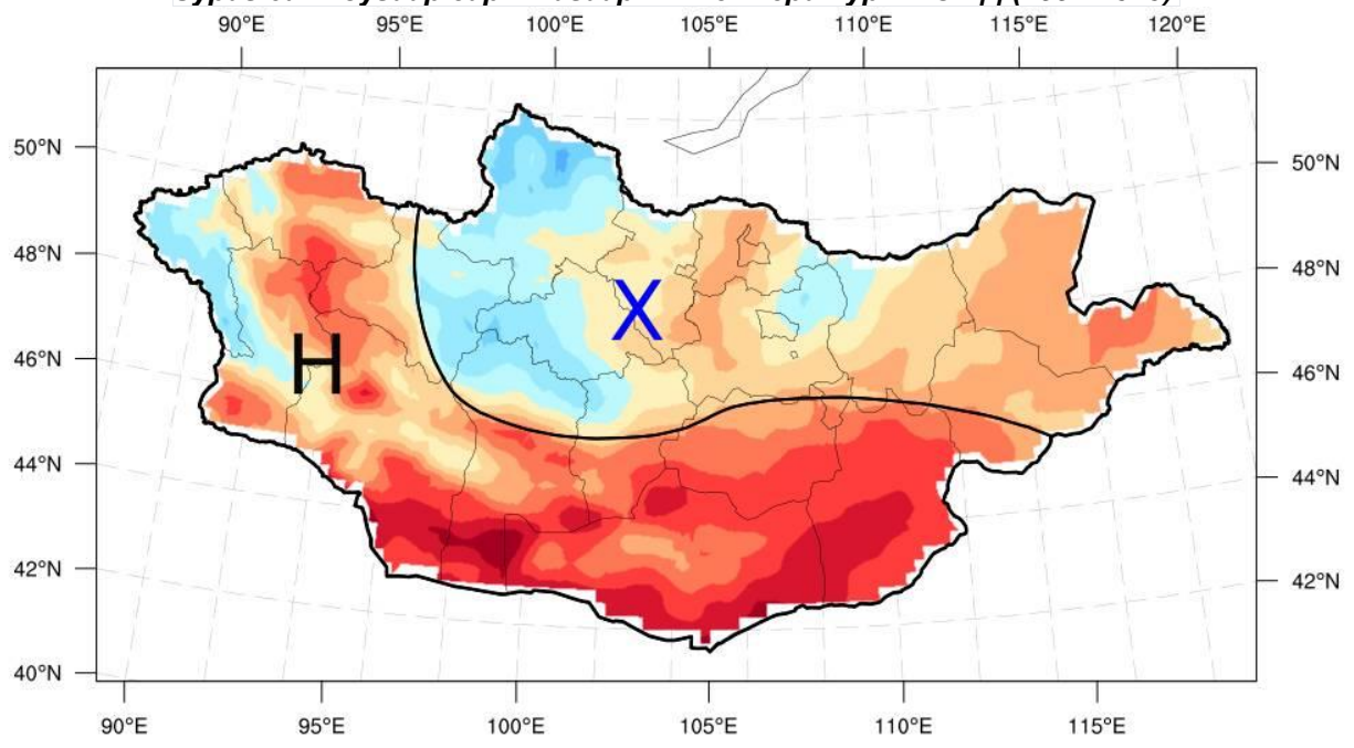
Зураг 5а. 7 дугаар сарын агаарын температурын ОЖД (1991-2020)
