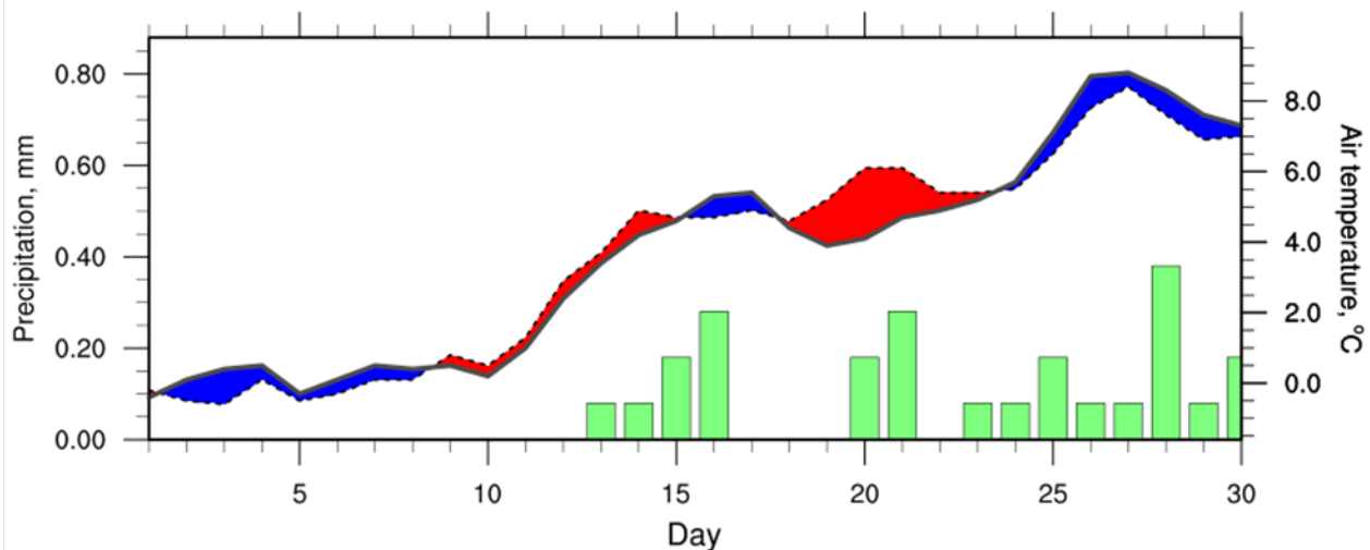
Зураг 6. Баруун аймгуудын нутгийн 2024 оны 04-р сарын агаарын температур, хур тунадасны явц [Үргэлжилсэн хар зураас – агаарын дундаж температурын ОЖД, тасархай хар зураас – агаарын дундаж температурын ОЖД-аас хазайх хазайц, улаан – агаарын дундаж температур ОЖД-аас дулаан, хөх – агаарын дундаж температур ОЖД-аас хүйтэн, ногоон – хур тунадасны хэмжээ]
