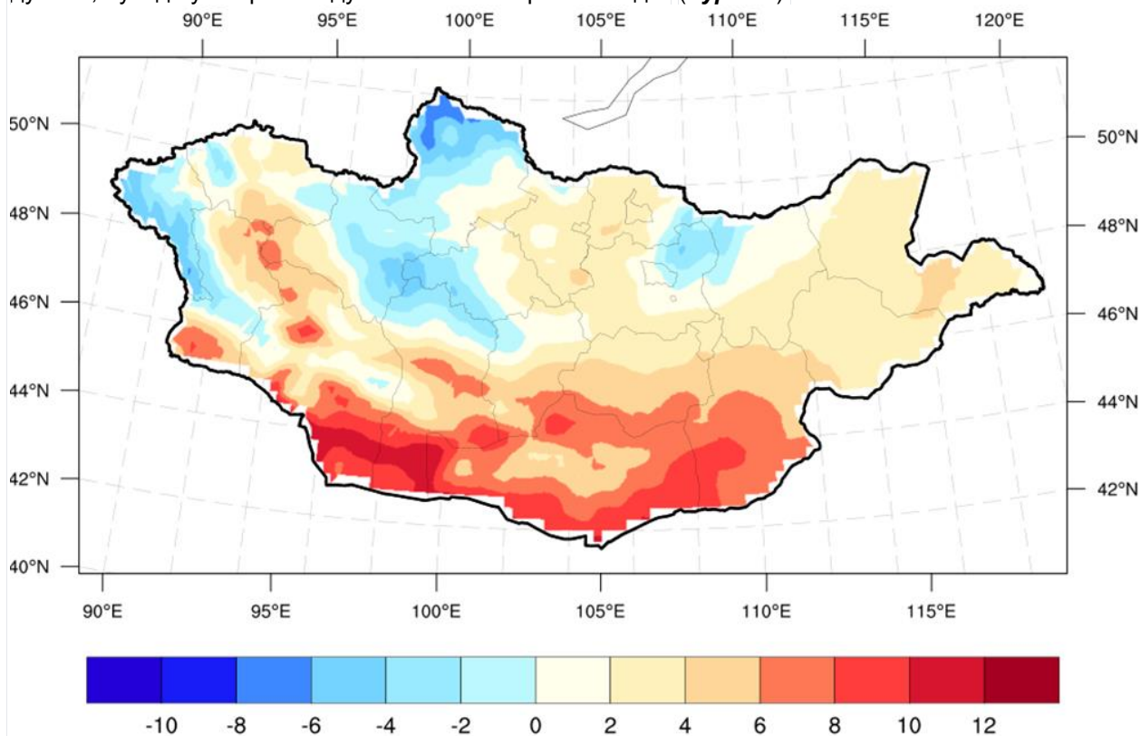
Зураг 1. 04-р сарын агаарын температурын ОЖД, [°C].
