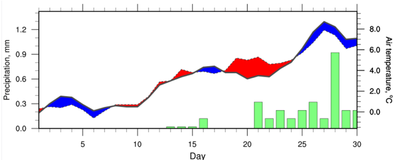
Зураг 7. Төвийн аймгуудын нутгийн 2024 оны 04-р сарын агаарын температур, хур тунадасны явц
