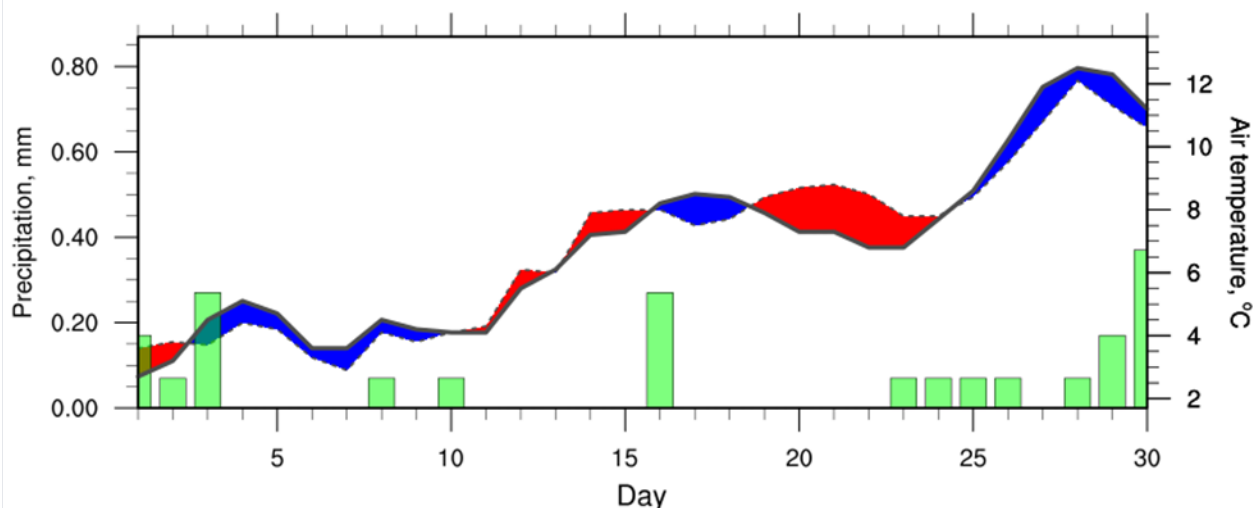
Зураг 9. Говийн аймгуудын нутгийн 2024 оны 04–р сарын агаарын температур, хур тунадасны явц
