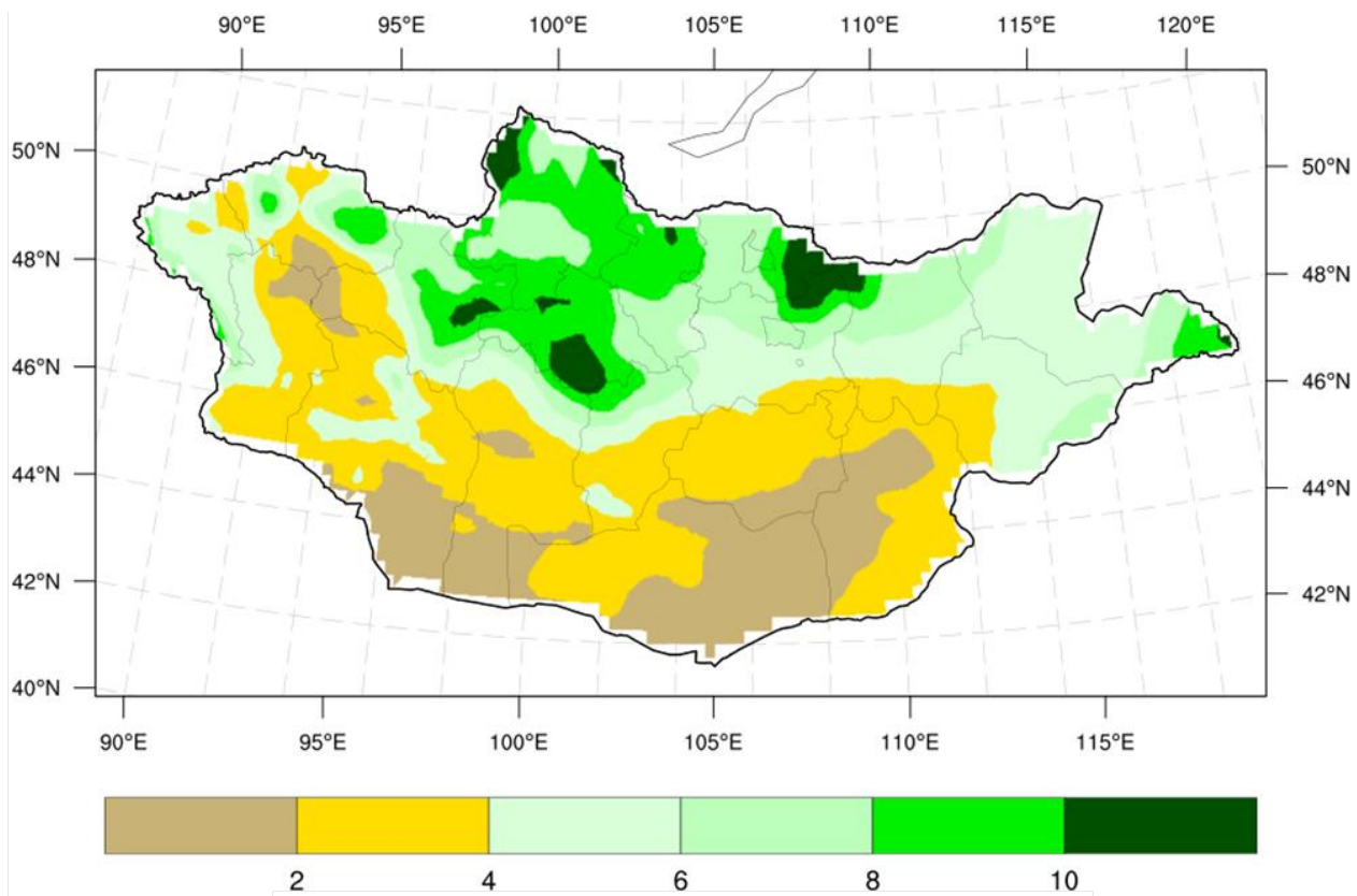
Зураг 2. 04-р сарын нийлбэр хур тунадасны ОЖД, [мм].
