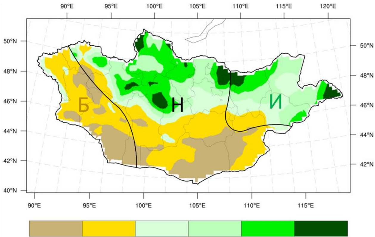
Зураг 5. 2024 оны 04-р сарын нийлбэр хур тунадасны урьдчилсан мэдээ, мм [И – хур тунадас ОЖД-аас их, Н – хур тунадас ОЖД-ийн орчим, Б – хур тунадас ОЖД – аас бага]
