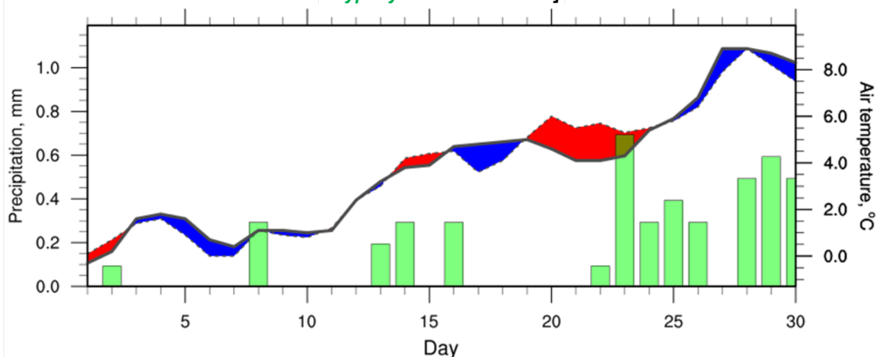
Зураг 8. Зүүн аймгуудын нутгийн 2024 оны 04-р сарын агаарын температур, хур тунадасны явц
