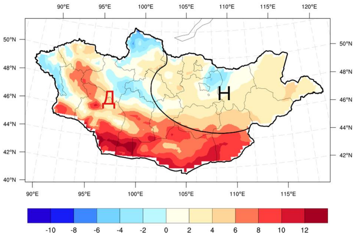
Зураг 4. 2024 оны 04–р сарын агаарын дундаж температурын урьдчилсан мэдээ, C° [Д – агаарын дундаж температур ОЖД–аас дулаан, Н – агаарын дундаж температур ОЖД–ийн орчим]
