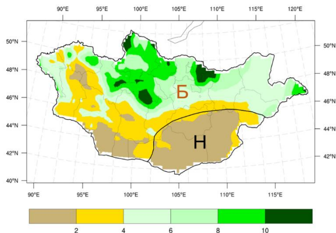
Зураг 6. 4 дүгээр сарын хур тунадасны урьдчилсан төлөв (мм) [Н – хур тунадас ОЖД–ийн орчим, Б – хур тунадас ОЖД–аас бага]
