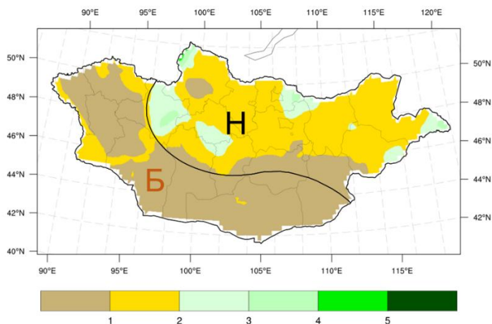
Зураг 2. 2 дугаар сарын хур тунадасны урьдчилсан төлөв (мм) [Н – хур тунадас ОЖД–ийн орчим, Б – хур тунадас ОЖД–аас бага]
