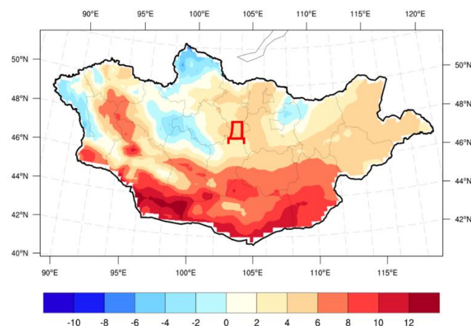
Зураг 5. 4 дүгээр сарын агаарын температурын урьдчилсан төлөв ( ^{\circ}\text{C} ) [Д – агаарын температур ОЖД–аас дулаан]
