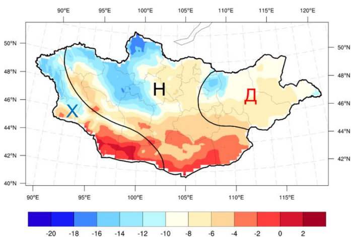
Зураг 3. 3 дугаар сарын агаарын температурын урьдчилсан төлөв (°C) [Д – агаарын температур ОЖД–аас дулаан, Н – агаарын температур ОЖД–ийн орчим] Х – агаарын температур ОЖД–аас хүйтэн]
