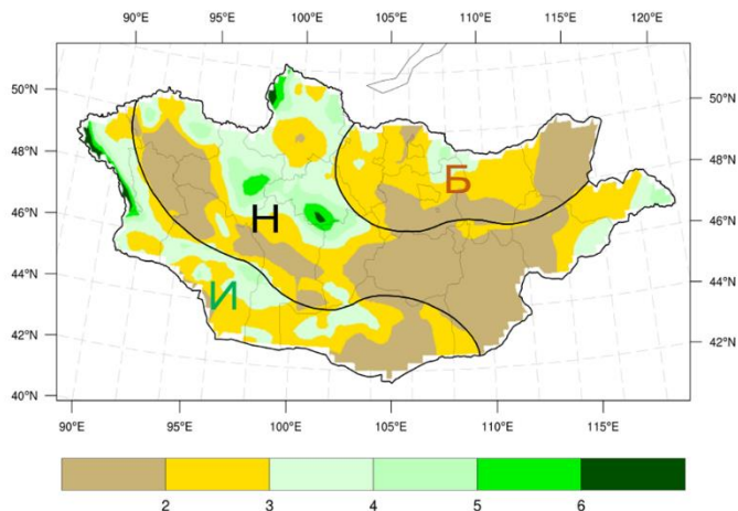
Зураг 4. 3 дугаар сарын хур тунадасны урьдчилсан төлөв (мм) [И–хур тунадас ОЖД–аас ахиу, Н – хур тунадас ОЖД–ийн орчим, Б – хур тунадас ОЖД–аас бага]
