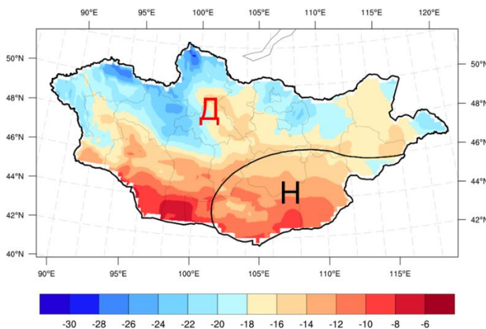
Зураг 1. 2 дугаар сарын агаарын температурын урьдчилсан төлөв (°C) [Д – агаарын температур ОЖД–аас дулаан, Н – агаарын температур ОЖД–ийн орчим]
