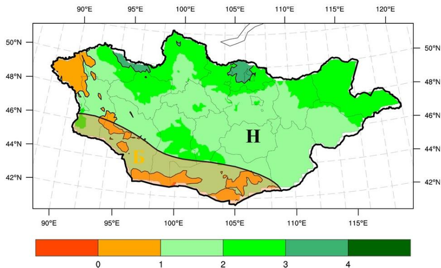
Зураг 6. 1 дүгээр сарын хур тунадасны урьдчилсан төлөв(мм)
