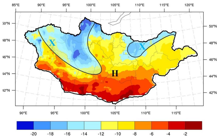
Зураг 1. 11 дүгээр сарын агаарын температурын урьдчилсан төлөв( ^{\circ}\text{C} )
