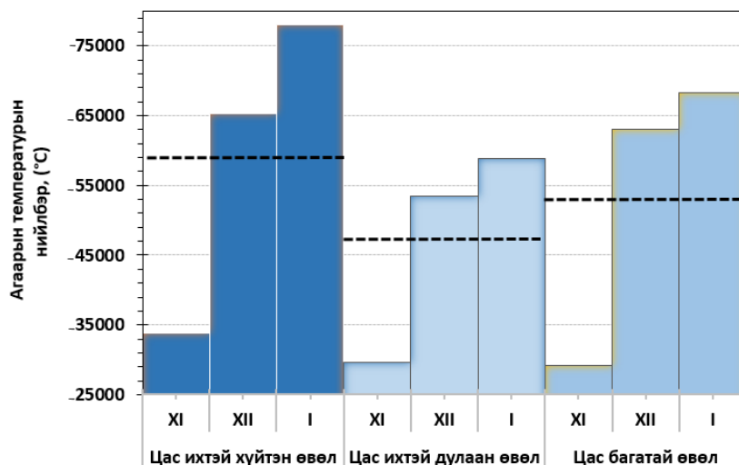
Зураг 7. Хүйтэн улирлын (12-1 сарын) цас ихтэй хүйтэн, цас ихтэй дулаан өвөл, цас багатай өвлийн улирлын агаарын хасах температурын (°C) нийлбэр (1981-2019). Тасархай хар шугам дунджийг илэрхийлэв.
