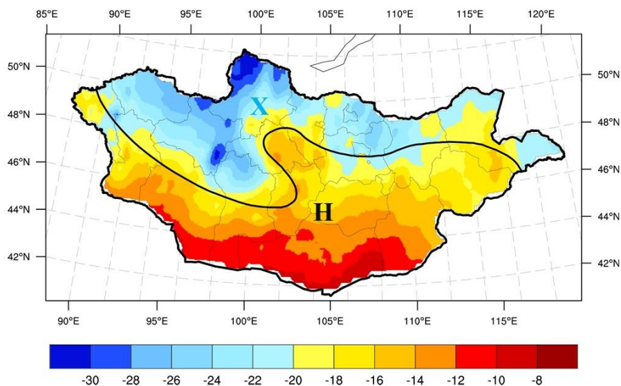
Зураг 3. 12 дугаар сарын агаарын температурын урьдчилсан төлөв(°C)
