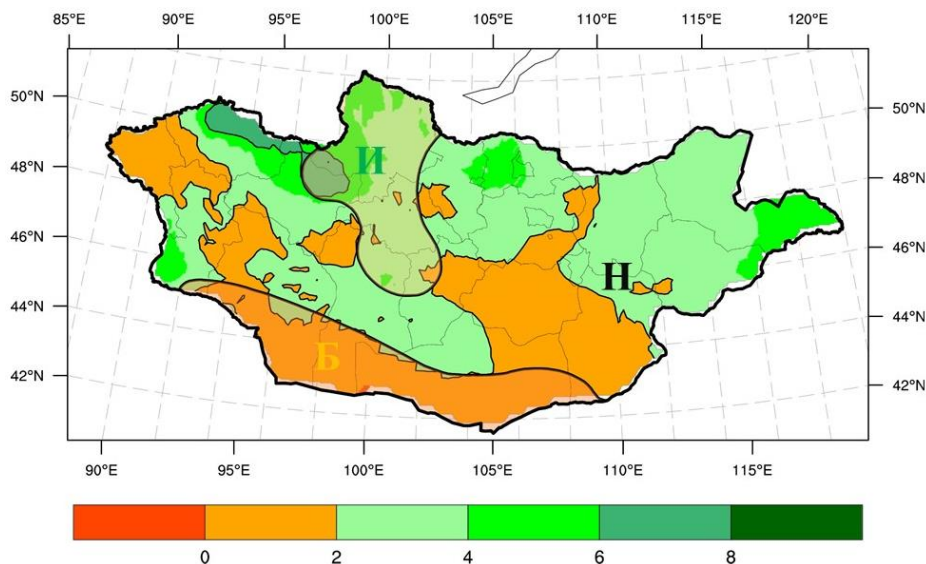
Зураг 4. 12 дугаар сарын хур тунадасны урьдчилсан төлөв(мм)
