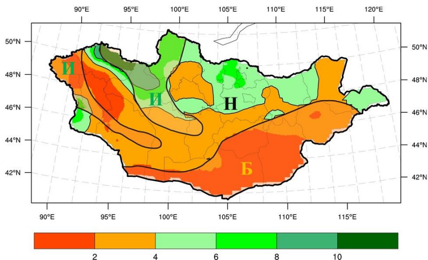
Зураг 2. 11 дүгээр сарын хур тунадасны урьдчилсан төлөв(мм)
