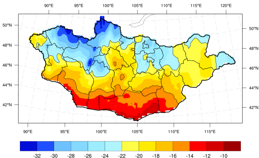
Зураг 5. 1 дүгээр сарын агаарын температурын урьдчилсан төлөв(°C)
